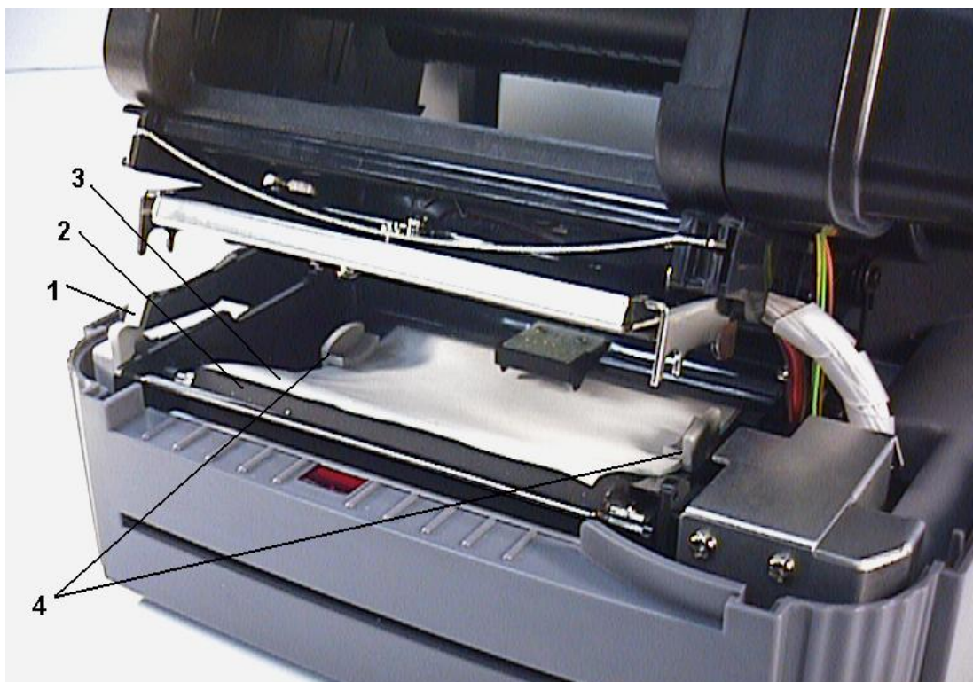
Рис. 6. Подача этикеток через регулируемую направляющую
