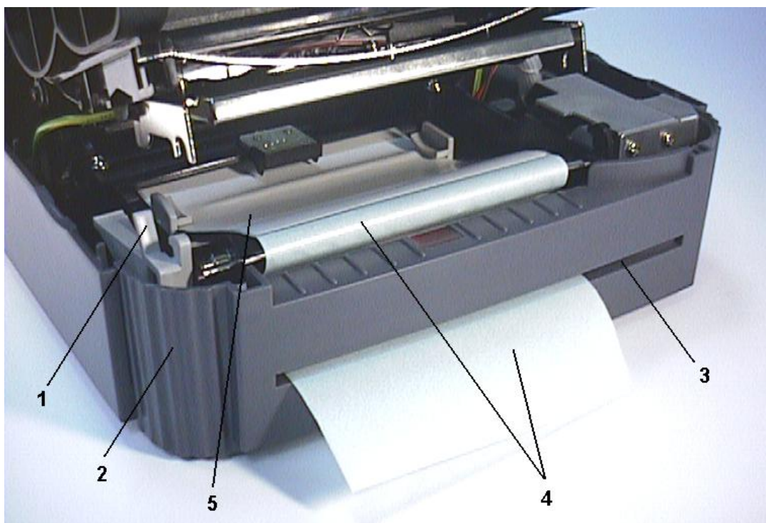
Рис. 8. Принтер подготовлен для работы с функцией автоотделения
